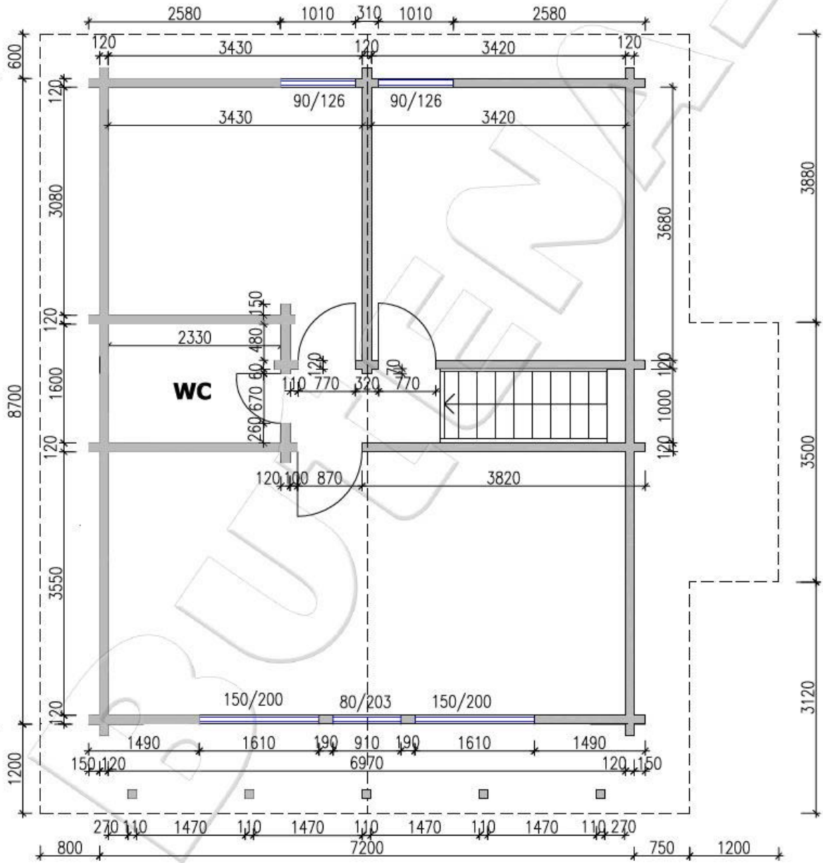
Grundriss 2
