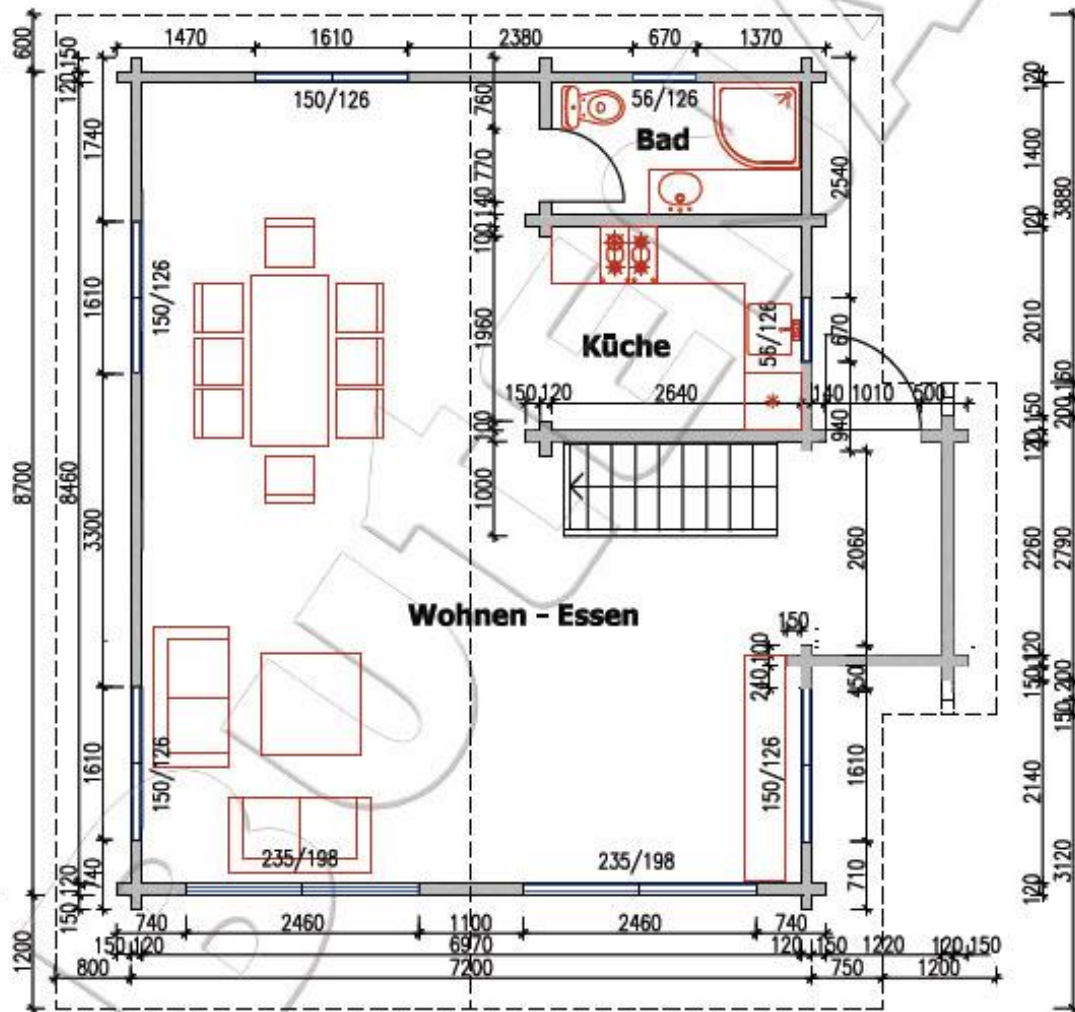
Grundriss 1
